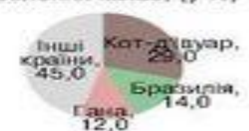
Мал. 53. Технічні культури світу (цукристі й тонізуючі)
