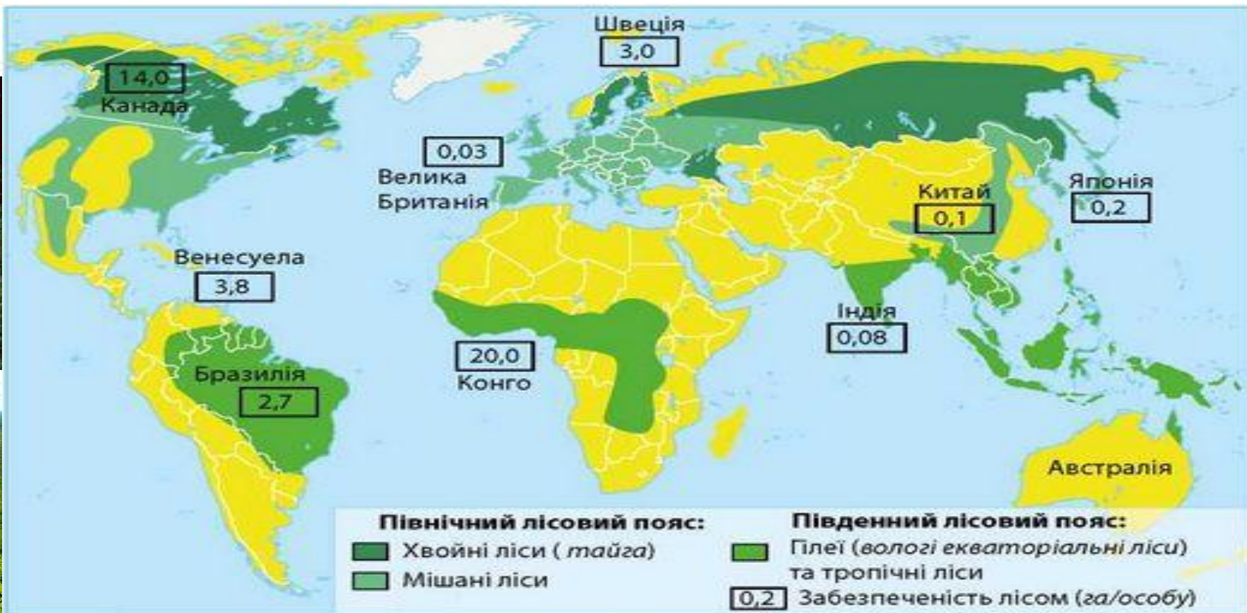
Мал. 58. Основні лісові пояси світу
